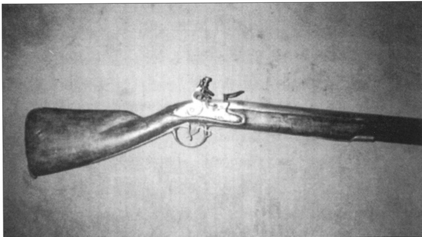
Русская фузья, сконструированная по австрийскому образцу 1754 г. Русская фузья выгодно отличалась от австрийского прототипа усиленной пружиной замка и металлическим шомполом вместо деревянного. Экземпляр из Государственного Исторического музея в Москве.
