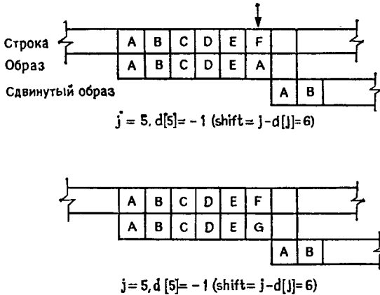
Рис. 1.12. Образ сдвигается за его последний символ.
