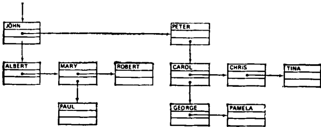
Рис. 4.43. Сильно ветвящееся дерево, представленное в виде двончного.
