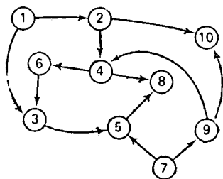
Рис. 4.13. Частично упорядоченное множество.
