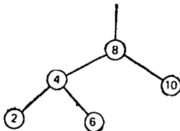
Рис. 4.31. Сбалансированное дерево.
