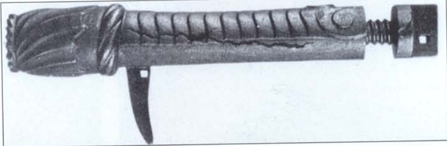
Сохранилось очень мало образцов средневекового ручного огнестрельного оружия. Данный образец - редкое исключение. Украшенный ствол этой ручной кулеврины при выстреле расширялся и имеет длинную продольную трещину. Крюк под стволом предназначался для того, чтобы при обороне замка цепляться за стену. Таким образом гасился откат орудия.
