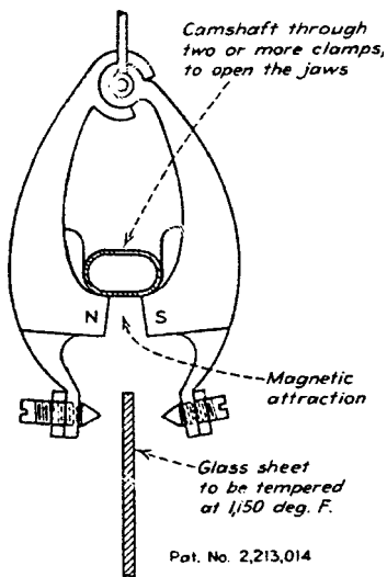
Fig. 7 A clamp.
