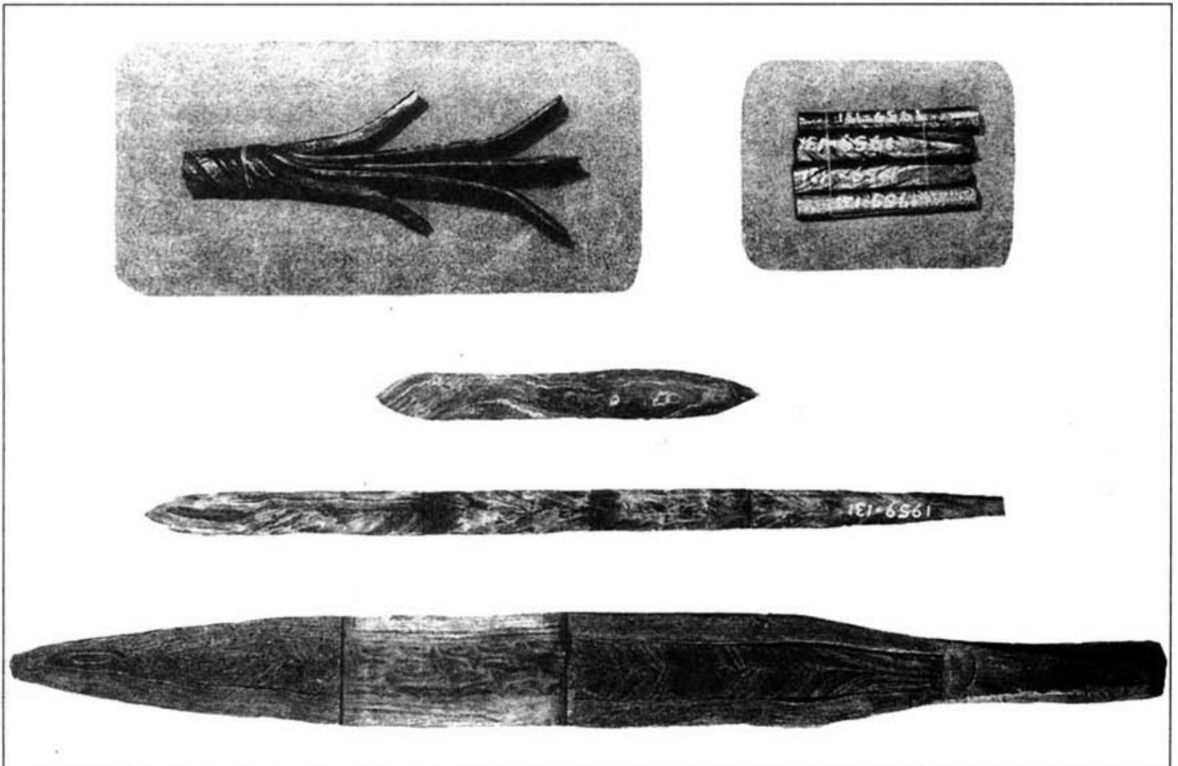
Стадии изготовления меча методом сварки. В верхнем левом углу показан пучок железных полос, скрученных жгутом и кованых молотом. Получившиеся в результате спиралевидные чушки показаны в правом верхнем углу. Группы таких чушек скручивались снова и опять ковались молотом, образуя сердечник меча. Наконец, к сердечнику добавлялись лезвия и коническая втулка. Центральная часть меча отполирована, чтобы дать представление об окончательном облике меча.
